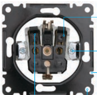
Механизмы розеток поставляются и с пружинным креплением кабеля
