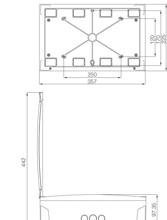
Корпус 16М наружной установки
