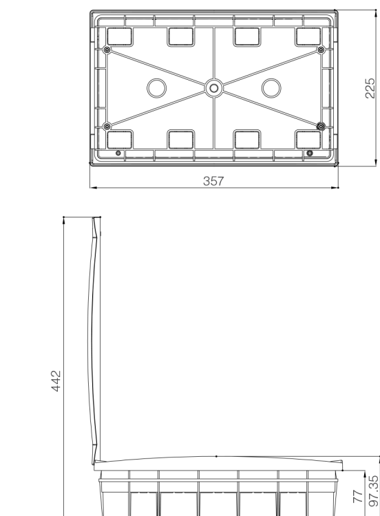
Корпус 16М внутренней установки
