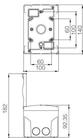
Корпус 2М наружной установки
