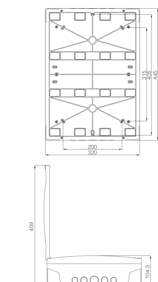
Корпус 36М наружной установки трех слойный
