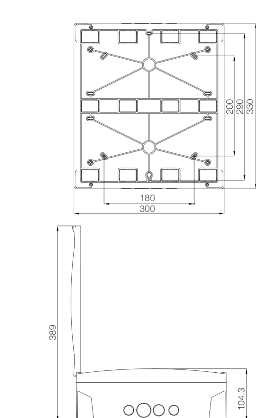
Корпус 24М наружной установки 2-х уровневый
