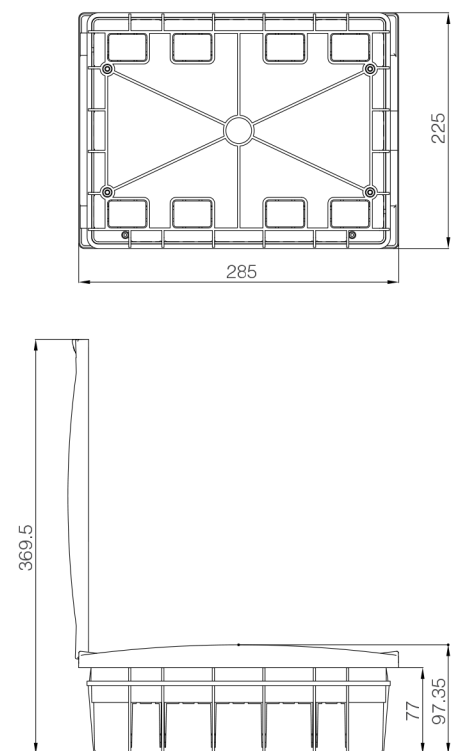
Корпус 12М внутренней установки
