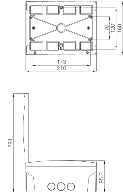
Корпус 8М наружной устаовки
