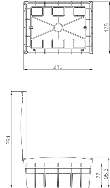
Корпус 8М внутренней установки
