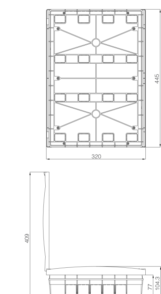
Корпус 36М внутренней установки трех слойный
