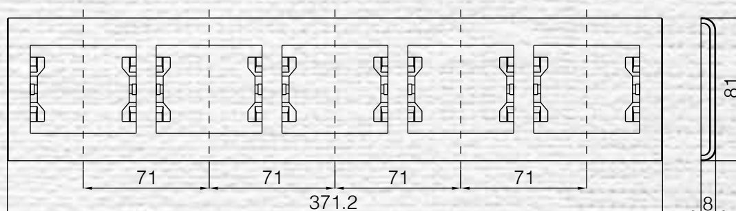
Рамка 5-я горизонтальная
