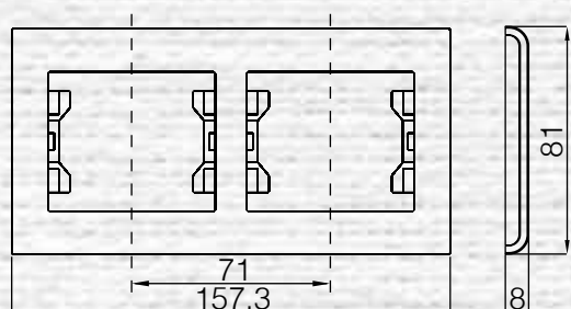
Рамка 2-я горизонтальная
