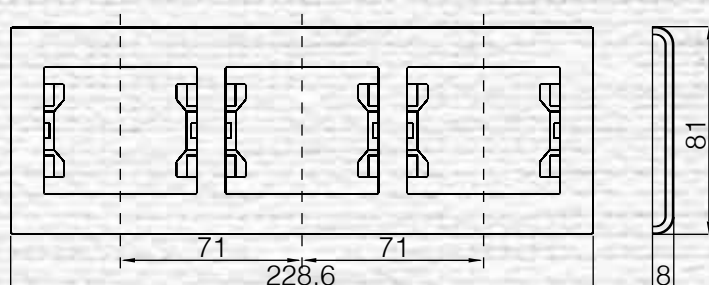
Рамка 3-я горизонтальная
