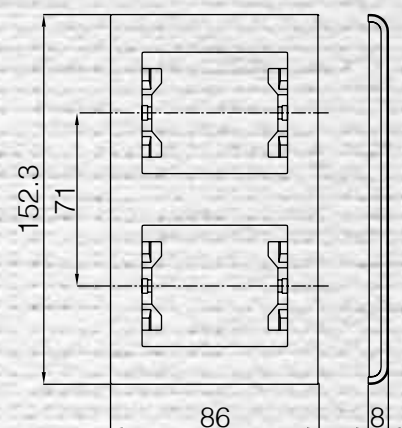
Рамка 2-я вертикальная
