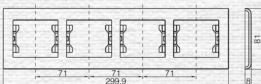
Рамка 4-я горизонтальная
