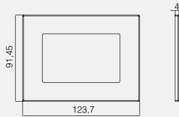
Kare 3M Frame
