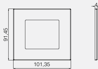
Kare 2M Frame
