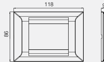
Millanta 3M Frame
