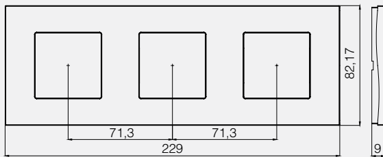
Kare 3x2M Frame
