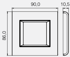
Cellia 2M Frame
