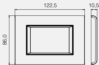
Cellia 3M Frame
