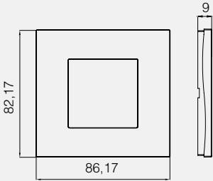
Kare 2M Frame
