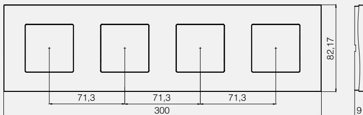
Kare 4x2M Frame
