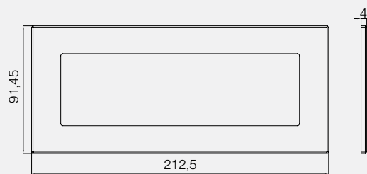
Kare 7M Frame
