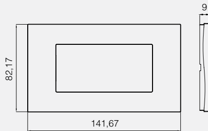
Kare 4M Frame
