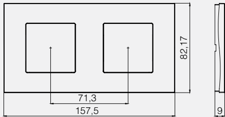
Kare 2x2M Frame
