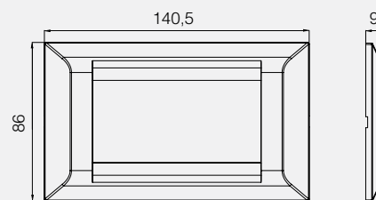
Millanta 4M Frame
