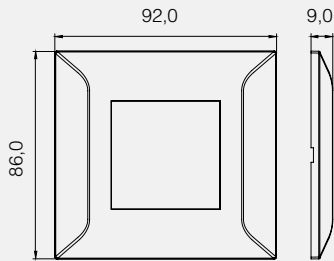
Millanta 2M Frame
