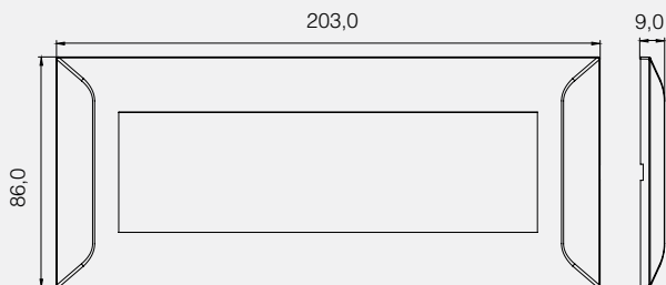
Millanta 7M Frame
