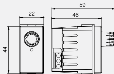
Vavien Dimmer 300 V
