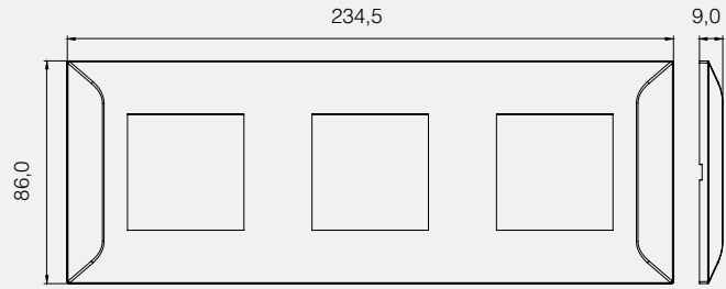
Millanta 3x2M Frame
