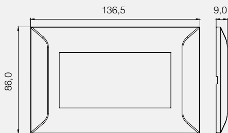
Millanta 4M Frame
