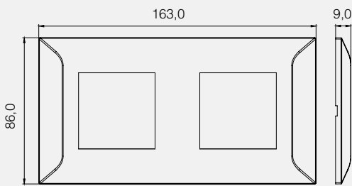
Millanta 2x2M Frame
