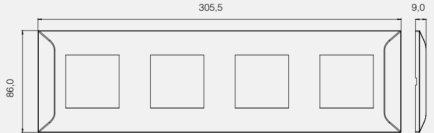
Millanta 4x2M Frame
