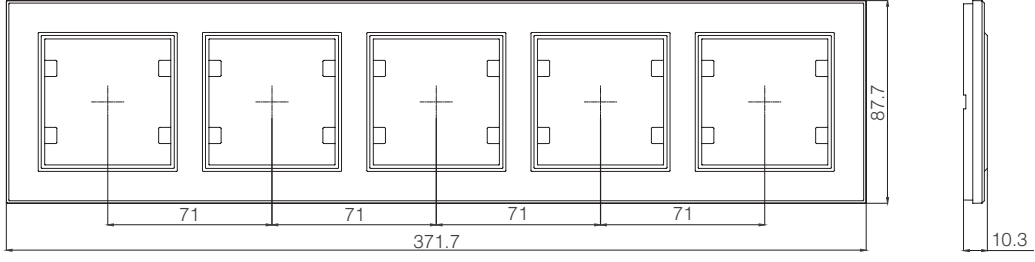
Beşli Yatay Çerçeve
