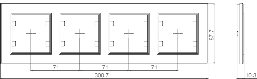
Dörtlü Yatay Çerçeve
