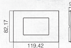
3M рамка / 3M Frame
