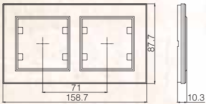
Рамка 2-я горизонтальная / Double Horizontal Frame
