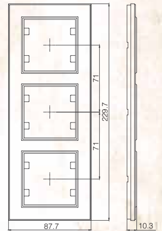
Рамка 3-я вертикальная Triple Vertical Frame
