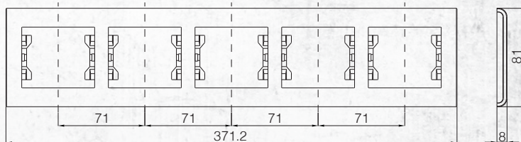
Рамка 5-я горизонтальная / Fiftet Horizontal Frame
