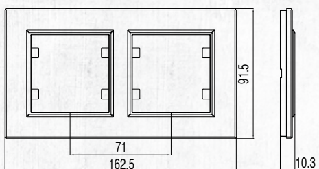
Рамка 2-я горизонтальная Double Horizontal Frame
