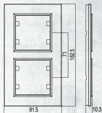
Рамка 2-я вертикальная Double Vertical Frame
