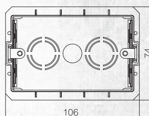
Монтажная коробка 3М 3M Flush Mounted cases
