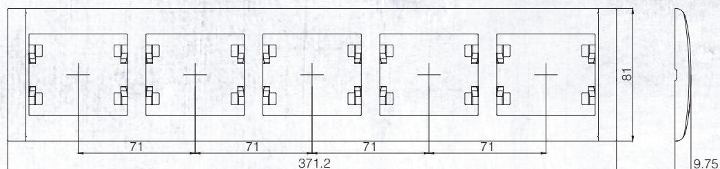
Рамка 5-я горизонтальная / Fiftet Horizontal Frame
