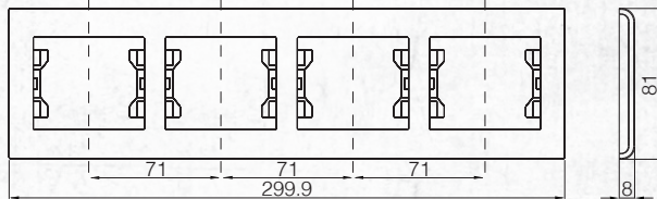
Рамка 4-я горизонтальная / Quartet Horizontal Frame
