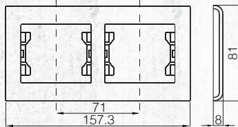
Рамка 2-я горизонтальная / Double Horizontal Frame
