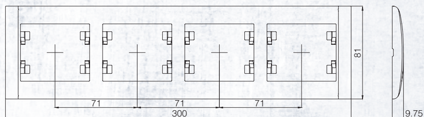
Рамка 4-я горизонтальная / Quartet Horizontal Frame
