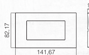
4M рамка / 4M Frame
