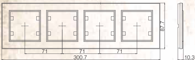
Рамка 4-я горизонтальная / Quartet Horizontal Frame
