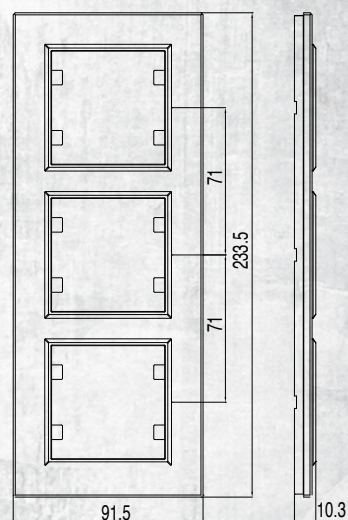
Рамка 3-я вертикальная Triple Vertical Frame
