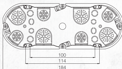
Монтажная коробка 7М 7M Cavity wall Case
