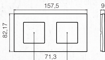
2x2M рамка / 2x2M Frame
