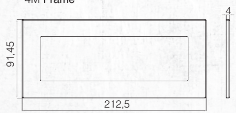
7M рамки 7M Frame
