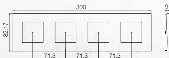
4x2M рамка / 4x2M Frame
