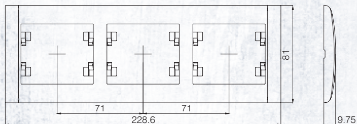
Рамка 3-я горизонтальная / Triple Horizontal Frame
