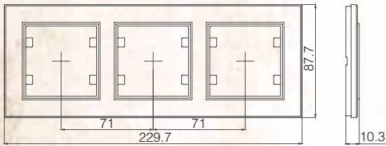
Рамка 3-я горизонтальная / Triple Horizontal Frame
