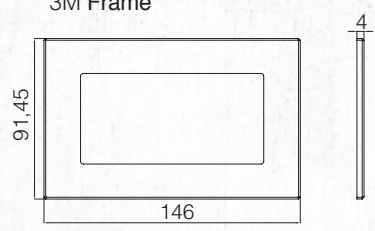
4M рамки 4M Frame
