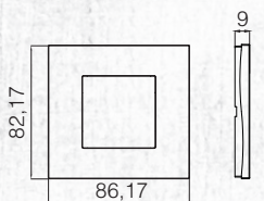
2M рамка / 2M Frame
