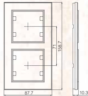
Рамка 2-я вертикальная Double Vertical Frame
