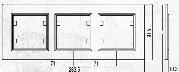
Рамка 3-я горизонтальная Triple Horizontal Frame
