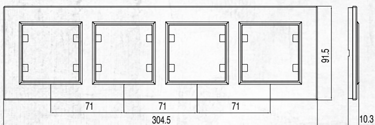
Рамка 4-я горизонтальная Quartet Horizontal Frame
