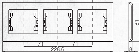
Рамка 3-я горизонтальная / Triple Horizontal Frame
