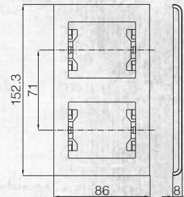
Рамка 2-я вертикальная Double Vertical Frame
