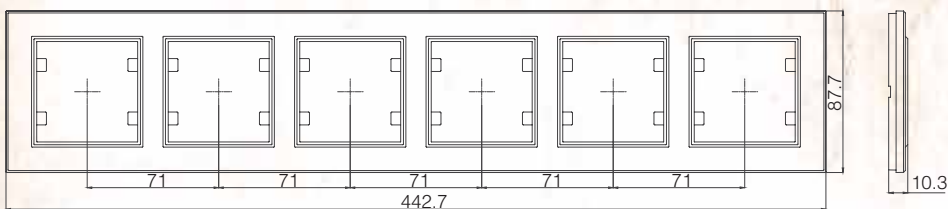
Рамка 6-я горизонтальная / Sixtet Horizontal Frame
