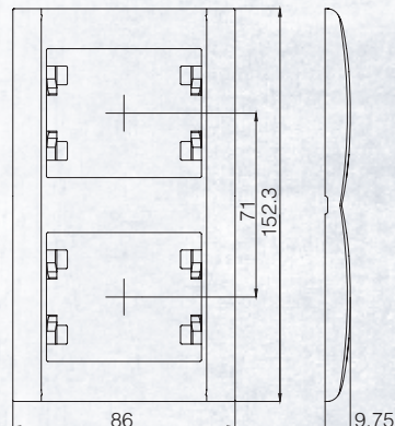
Рамка 2-я вертикальная Double Vertical Frame
