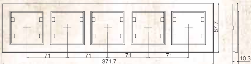
Рамка 5-я горизонтальная / Fiftet Horizontal Frame
