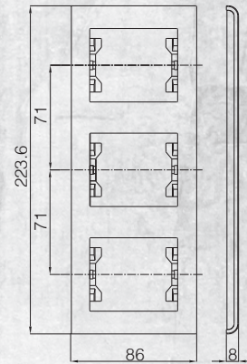
Рамка 3-я вертикальная Triple Vertical Frame
