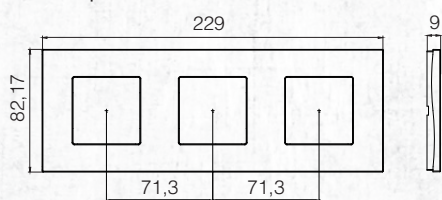
3x2M рамка / 3x2M Frame
