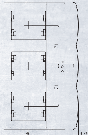
Рамка 3-я вертикальная Triple Vertical Frame
