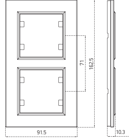
İkili Dikey Çerçeve Double Vertical Frame
