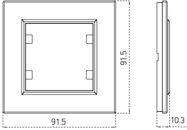
Tekli Çerçeve / Frame
