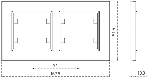
İkili Yatay Çerçeve / Double Horizontal Frame
