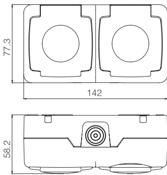
İkili Kapaklı Topraklı Priz
