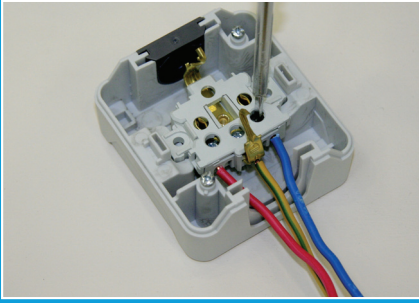
Vidalı bağlantı With screw terminals
