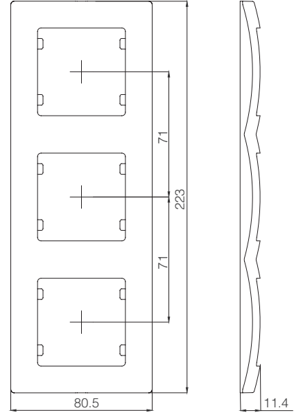
Üçlü Dikey Çerçeve
