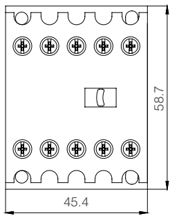
DC Mini Kontaktörler K09
