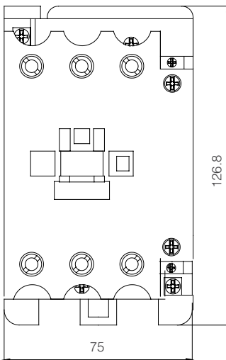
DC 24V Kontaktör 65A
