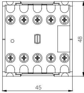
DC Mini Kontaktörler M06
