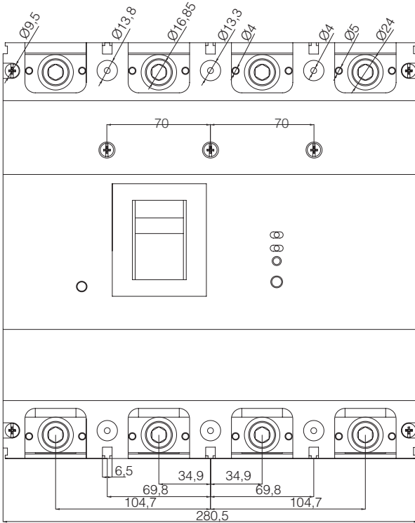
500 A, 630 A, 800 A Kaçak Akım Korumalı Kompakt Şalter
