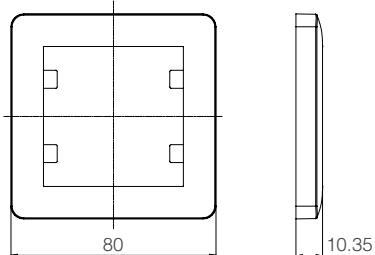
Рамка 1-я
