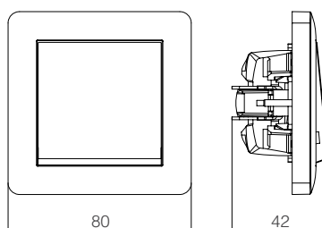
Выключатель одноклавишный
