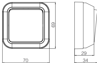
Выключатель одноклавишный
