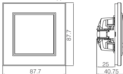
Выключатель одноклавишный
