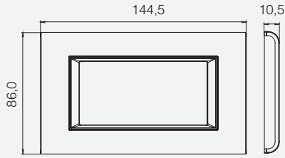
Cellia 4M Çerçeve
