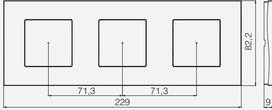
Kare 3x2M Çerçeve
