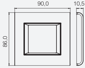
Cellia 2M Çerçeve
