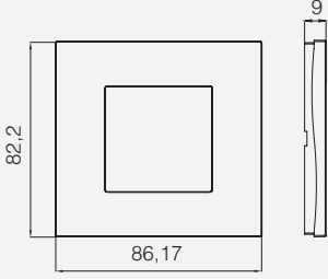
Kare 2M Çerçeve
