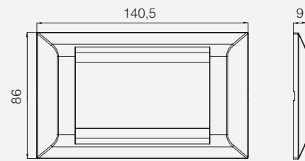
Millanta 4M Çerçeve
