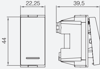
Anahtar / Işıklı Anahtar
