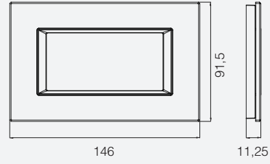
Kare 4M Çerçeve
