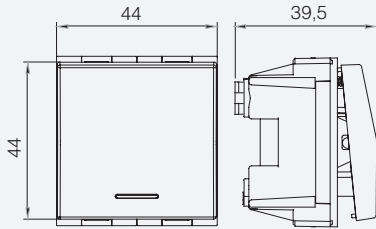
Anahtar / Işıklı Anahtar
