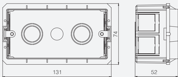
4M Sıva Altı Kasalar
