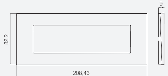
Kare 7M Çerçeve
