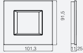
Kare 2M Çerçeve
