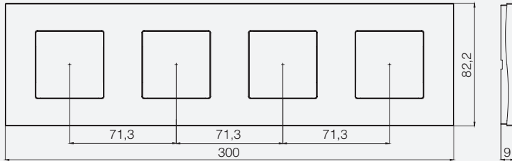
Kare 4x2M Çerçeve
