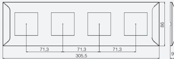
Millanta 4x2M Çerçeve
