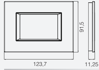
Kare 3M Çerçeve
