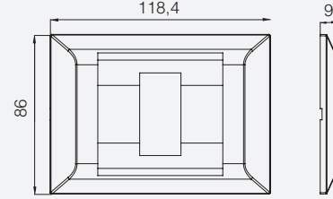
Millanta 1M Çerçeve (3M Boyutunda)
