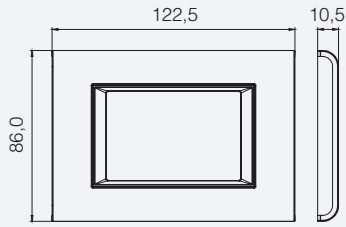
Cellia 3M Çerçeve
