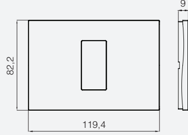
Kare 1M Çerçeve (3M Boyutunda)
