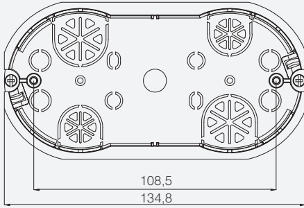
4M Alçıpan Kasa
