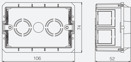
3M Sıva Altı Kasalar
