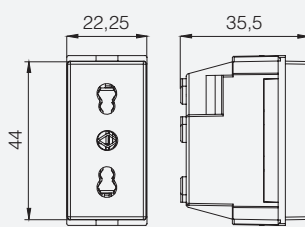
İtalyan Tipi Çocuk Korumalı Priz
