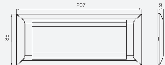
Millanta 7M Çerçeve
