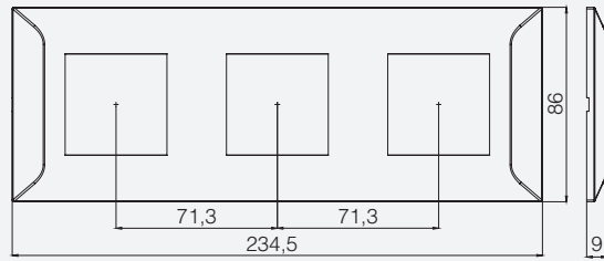
Millanta 3x2M Çerçeve
