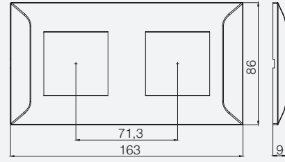
Millanta 2x2M Çerçeve
