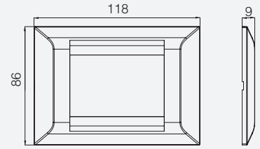
Millanta 3M Çerçeve
