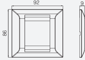
Millanta 2M Çerçeve
