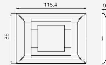
Millanta 2M Çerçeve (3M Boyutunda)
