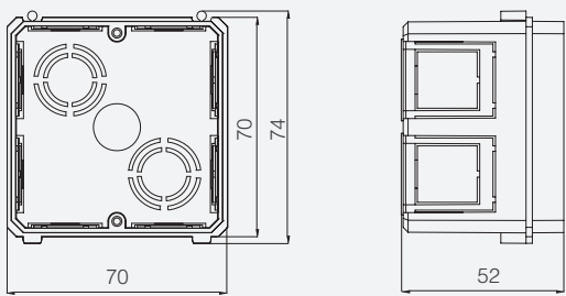
3M Sıva Altı Kasalar
