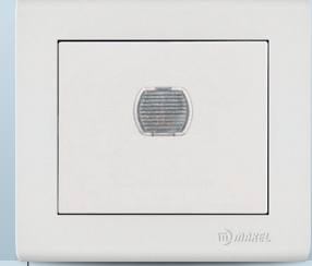
UZAKTAN KUMANDALI ŞEBEKE FİLTRELİ DİMMER REMOTE CONTROLLED TOROIDAL DIMMER 41001045 Çalışma Aralığı / Power Range 60W-600W Gerilim / Rated Voltage 250 V Koruma Derecesi / Protection IP20
