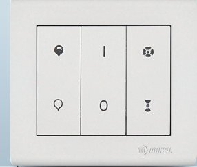
ÜÇLÜ KLİMA ANAHTARI COOLER SWITCH 41001084 Gerilim / Rated Voltage 250 V Akım / Rated Current 16 A Koruma Derecesi / Protection IP20
