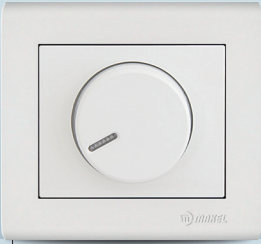
ŞEBEKE FİLTRELİ DİMMER TOROIDAL DIMMER 41001031 Çalışma Aralığı / Power Range 60W-600W Gerilim / Rated Voltage 250 V Koruma Derecesi / Protection IP20
