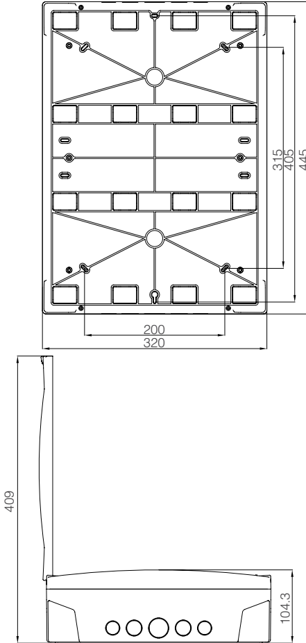
36'lı Sıva Üstü Klemensli Sigorta Kutusu
