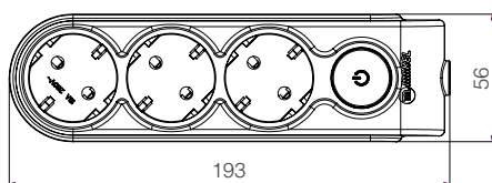
3Гн. Колодка с заземлением и выключателем
