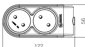
2Гн. Колодка с заземлением и выключателем
