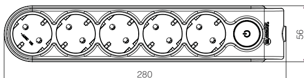
5Гн. Колодка с заземлением и выключателем
