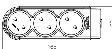
3Гн. Колодка с заземлением и выключателем
