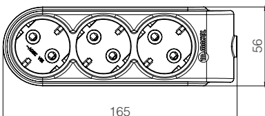
3Гн. Колодка с заземлением
