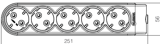
5Гн. Колодка с заземлением
