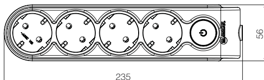
4Гн. Колодка с заземлением и выключателем
