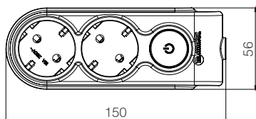
2Гн. Колодка с заземлением и выключателем
