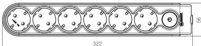
6Гн. Колодка с заземлением и выключателем
