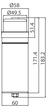
Tube Capacitor 5 (2,5 kVar)
