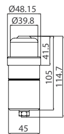
Tube Capacitor 1 (0,26 kVar)
