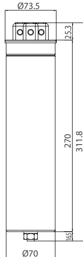
Tube Capacitor 9 (12,5 kVar)
