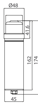
Tube Capacitor 2 (0,55-1-1,5 kVar)
