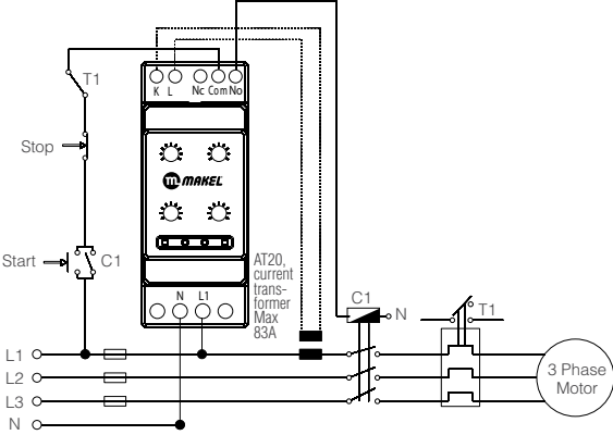
AKM-01T
