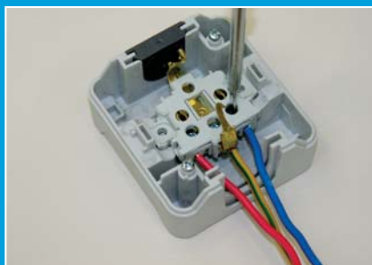
Винтовой зажим
