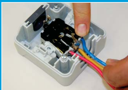
Пружинный зажим
