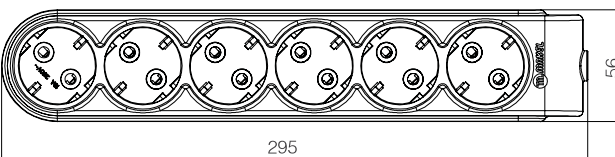
Altılı Topraklı Grup Priz
