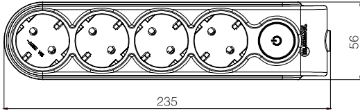
Dörtlü Topraklı Grup Priz Anahtarı
