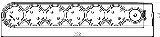
Altılı Topraklı Grup Priz Anahtarı
