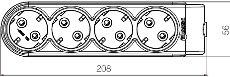
Dörtlü Topraklı Grup Priz
