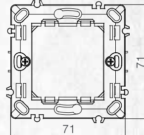
2M Tırnaklı Karkas
