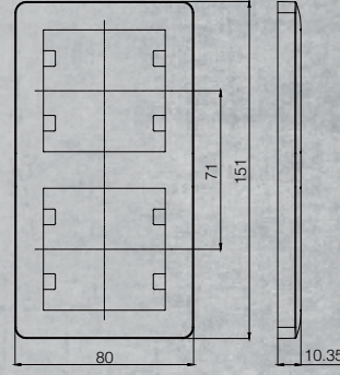
İkili Dikey Çerçeve
