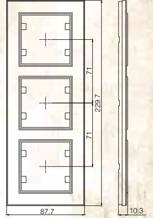
Üçlü Dikey Çerçeve
