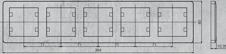
Beşli Yatay Çerçeve
