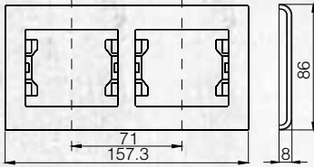
İkili Yatay Çerçeve
