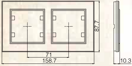
İkili Yatay Çerçeve
