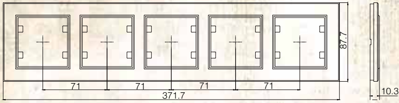
Beşli Yatay Çerçeve
