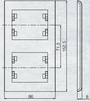
İkili Dikey Çerçeve
