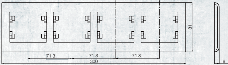
Dörtlü Yatay Çerçeve
