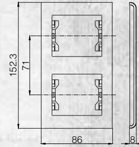
İkili Dikey Çerçeve
