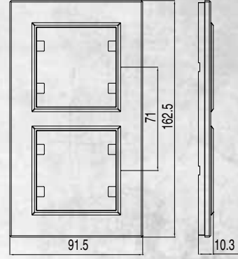
İkili Dikey Çerçeve
