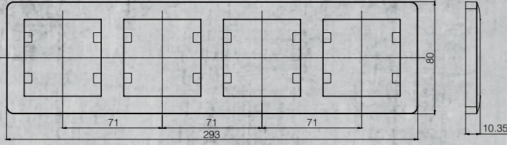
Dörtlü Yatay Çerçeve
