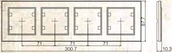
Dörtlü Yatay Çerçeve
