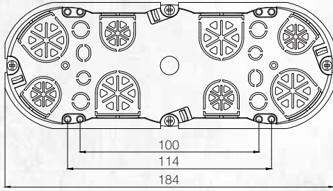
7M Alçıpan Kasa
