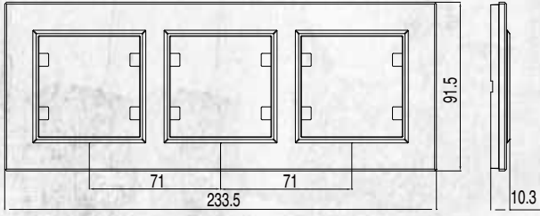
Üçlü Yatay Çerçeve
