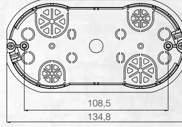
4M Alçıpan Kasa
