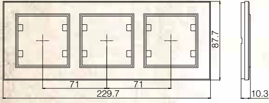
Üçlü Yatay Çerçeve
