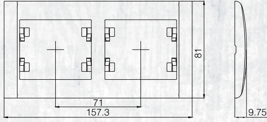
İkili Yatay Çerçeve
