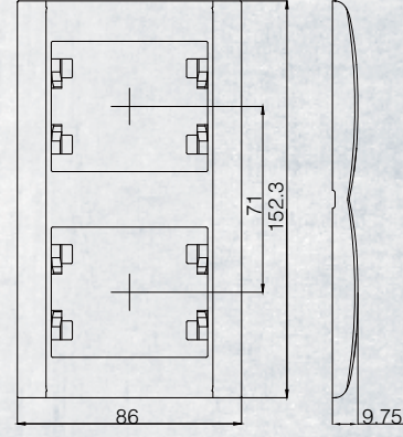
İkili Dikey Çerçeve
