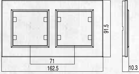
İkili Yatay Çerçeve
