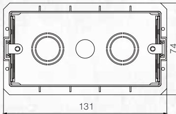
4M Sıva Altı Kasalar
