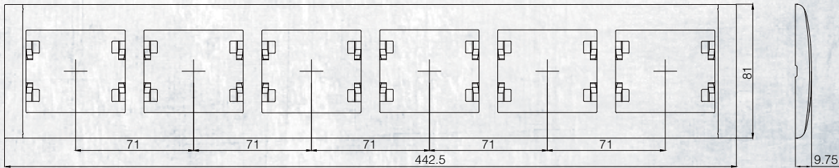
Altılı Yatay Çerçeve
