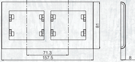
İkili Yatay Çerçeve
