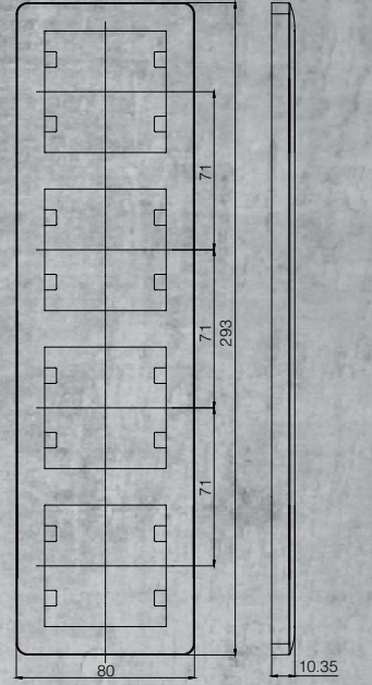
Dörtlü Dikey Çerçeve
