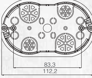
3M Alçıpan Kasa
