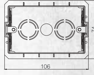
3M Sıva Altı Kasalar
