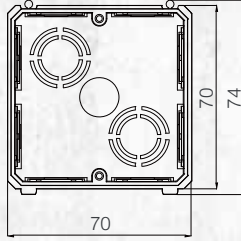
2M Sıva Altı Kasalar
