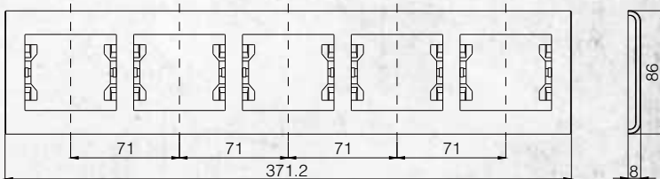
Beşli Yatay Çerçeve
