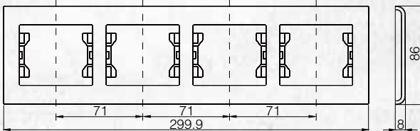
Dörtlü Yatay Çerçeve
