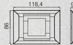
2M Çerçeve (3M Boyutunda)
