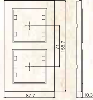
İkili Dikey Çerçeve
