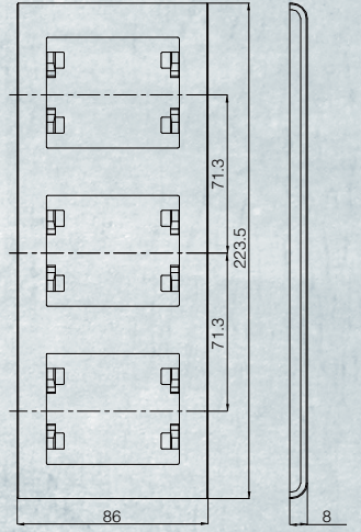
Üçlü Dikey Çerçeve
