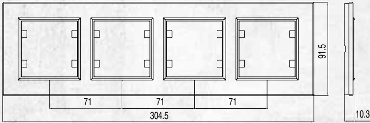
Dörtlü Yatay Çerçeve
