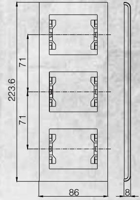
Üçlü Dikey Çerçeve
