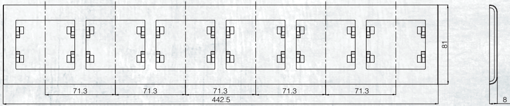
Altılı Yatay Çerçeve
