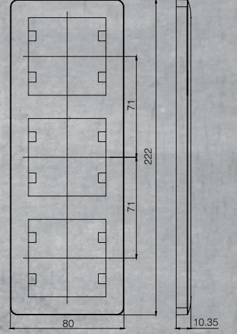
Üçlü Dikey Çerçeve
