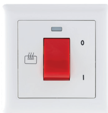
Heater Switch 45A BR016801 45 A, 250 V~ BS EN 60669-1
